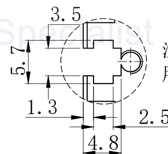
视图A
