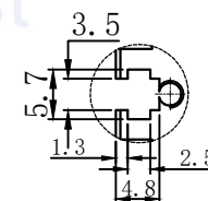
视图A
