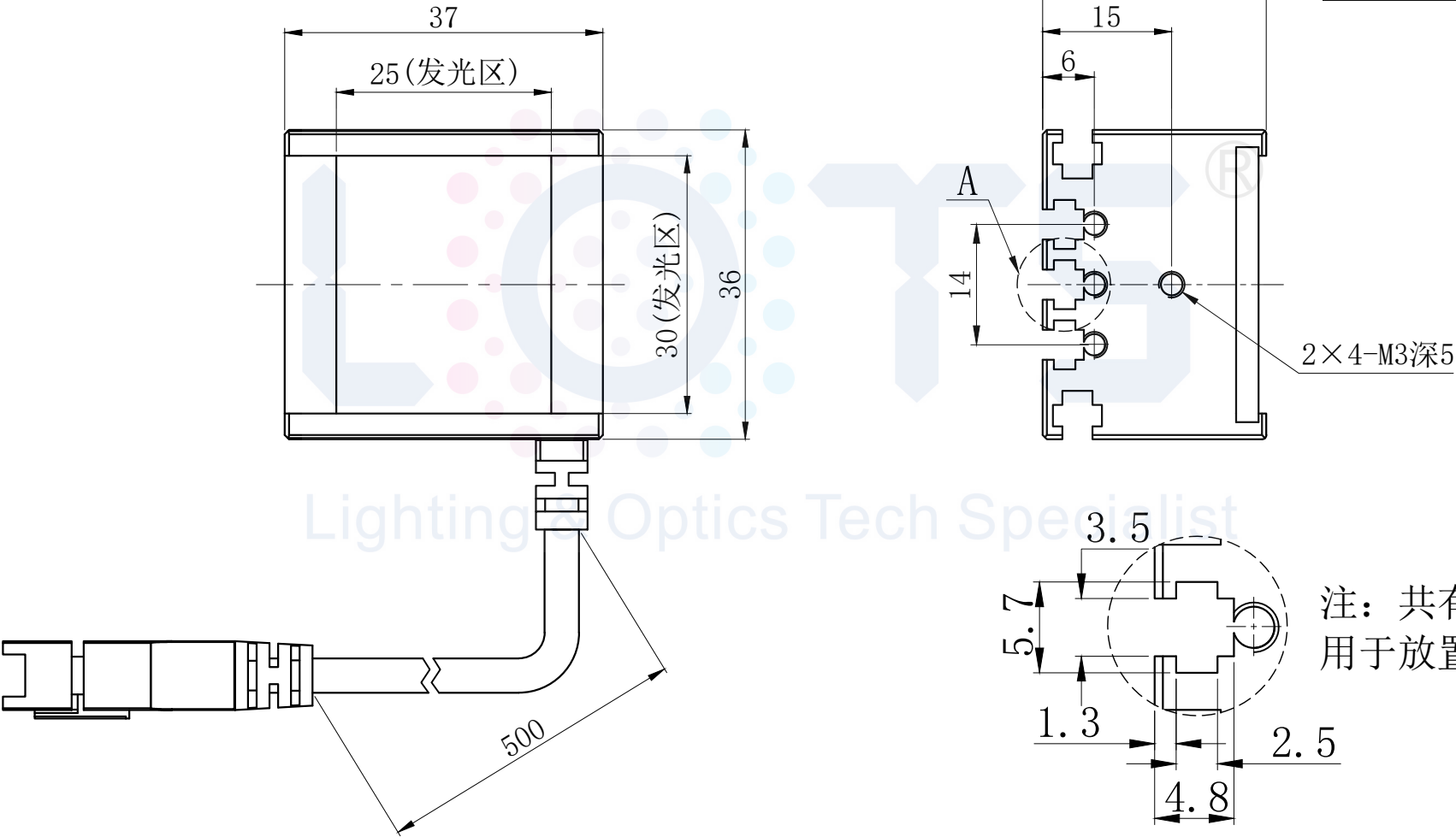
视图A
